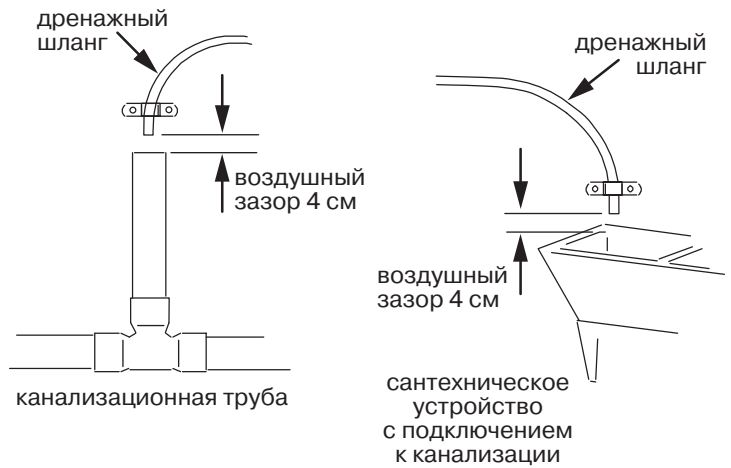
Подключение дренажа
